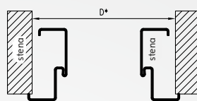
příčný řez s alternativním způsobem montáže
