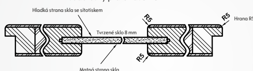
Vodorovný průřez dveří C1
