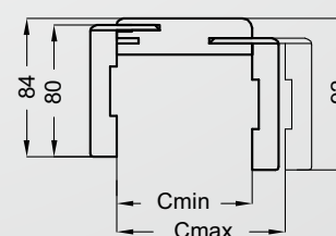
průřez T80
