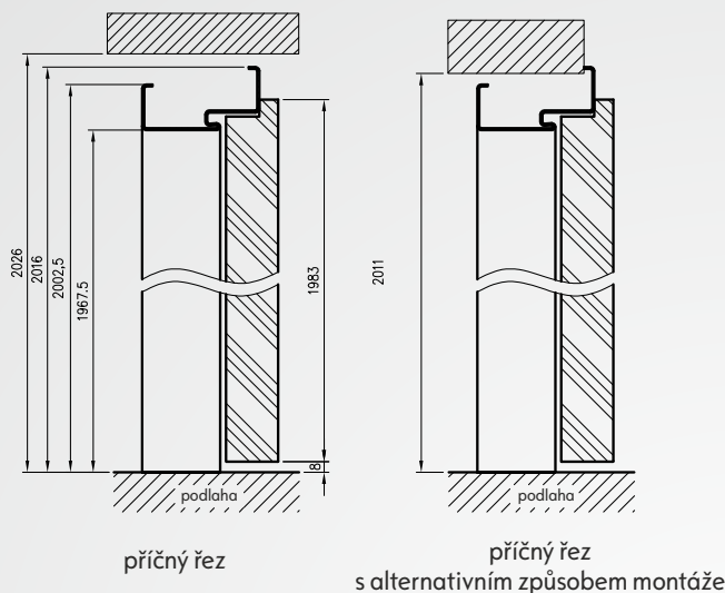
příčný řez s alternativním způsobem montáže
