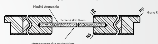
Vodorovný průřez dveří C5, C10
