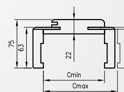
průřez T63
