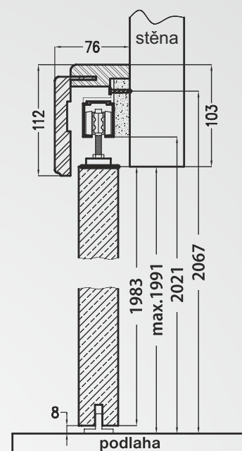
průřez posuvního systému NS
