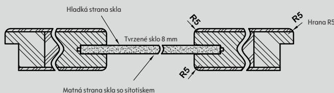
Vodorovný průřez dveří B5, B10 - B11
