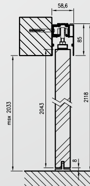
příčný řez
