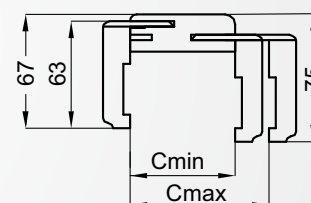
průřez K63
