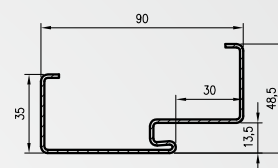
řez ocelovou zárubní
