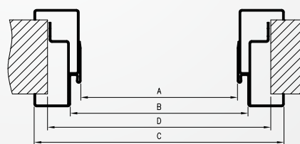
příčný řez s montážní kotvou
